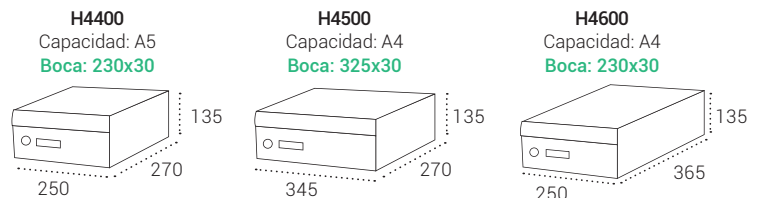
H4400-G3 Fondo 270 H4500-G3 Fondo 270 H4600-G3 Fondo 365
