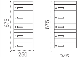
H4400-G5 Fondo 270 H4500-G5 Fondo 270 H4600-G5 Fondo 365
